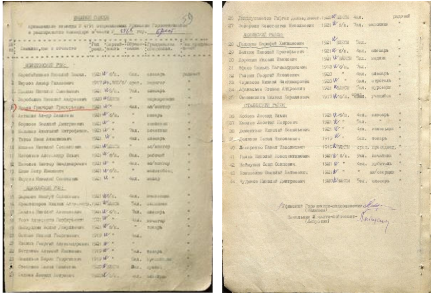
Рисунок 1. Список команды 4191
